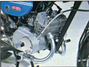
MOTEUR Tout nouveau bicylindre vertical à 5 lumières avec le système d'injection d'huile exclusif Yamaha Autolube.
